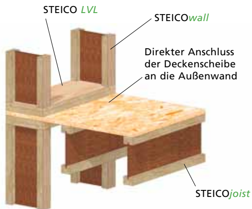
F3 Anschluss der Deckenscheibe zur Außenwand
