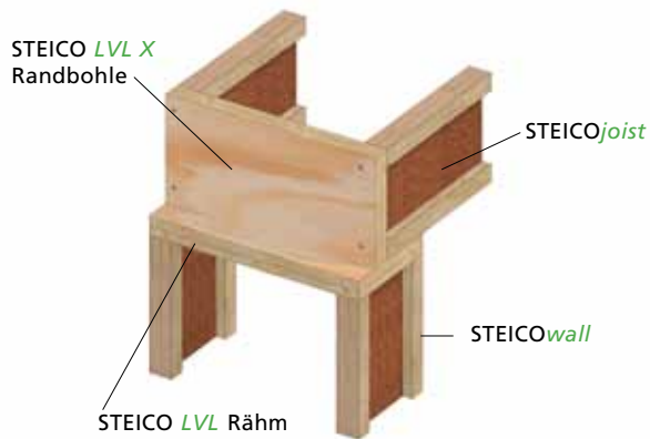
F1 Deckenanschluss mit Randbohle
